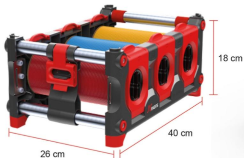
Sistema MOBIWAY™ POP
